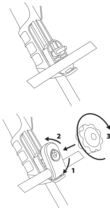
Ajuste del manillar en altura y posición
