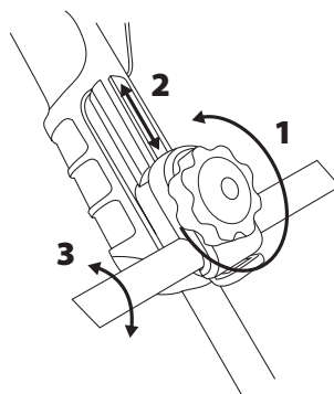
Réglage de la hauteur et de la position du guidon
