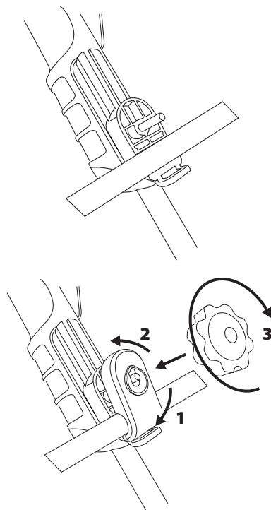
Réglage de la hauteur et de la position du guidon
